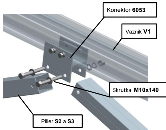
zoraďenie nosných pilierov "rámu" carportu
